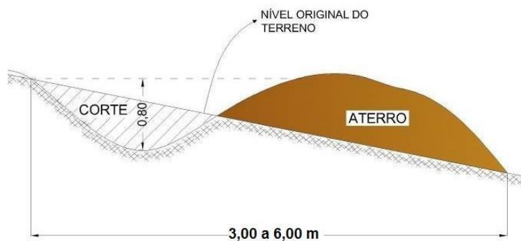
Figura 5. Esquema típico construção de terraço terração em nível.
