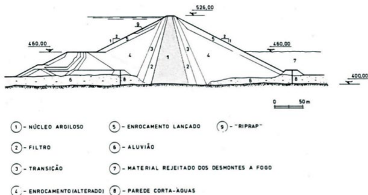
Figura 12. Seção típica de uma barragem de terra – enrocamento.
