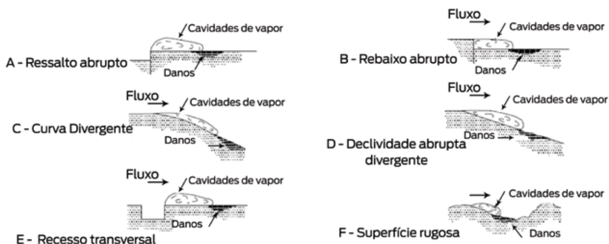
Figura 40. Tipos de irregularidades de superfícies de concreto e zonas de erosão por cavitação. Fonte: INAG, 2001
