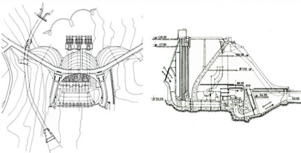
Figura 25. Barragem da Aguieira, Portugal (arcos múltiplos de grandes vãos de dupla curvatura, com 89 m de altura máxima, concluída em 1981). Fonte: CNPGB, 1992 / Banco de Imagens ANA
