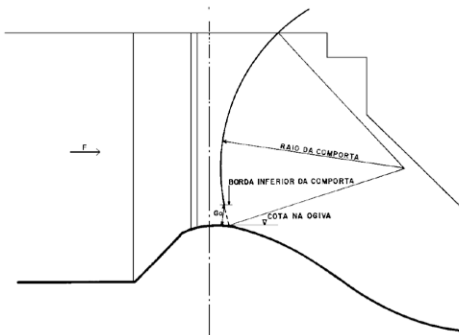
Figura 31. Eixo e viga de apoio das comportas. Fonte: ELETROBRAS, 2003, Figura 3.2
