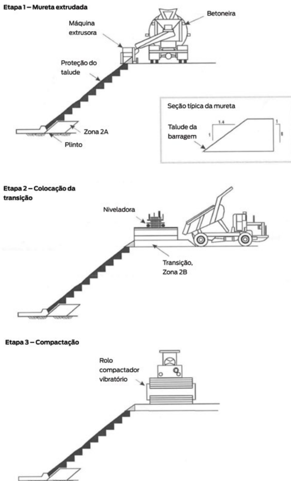
Figura 18. Construção da borda do talude de montante com material 2A. Fonte: ICOLD, 2010
