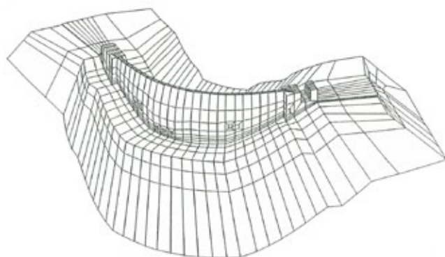
Modelo de elementos finitos– vista de montante
