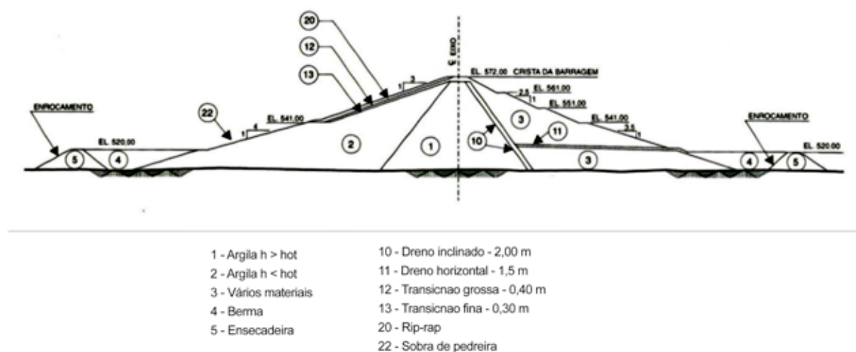
Figura 11. Seção típica de uma barragem de terra zonada. Barragem de Três Marias, MG – seção no leito do rio. Fonte: CRUZ, 2004
