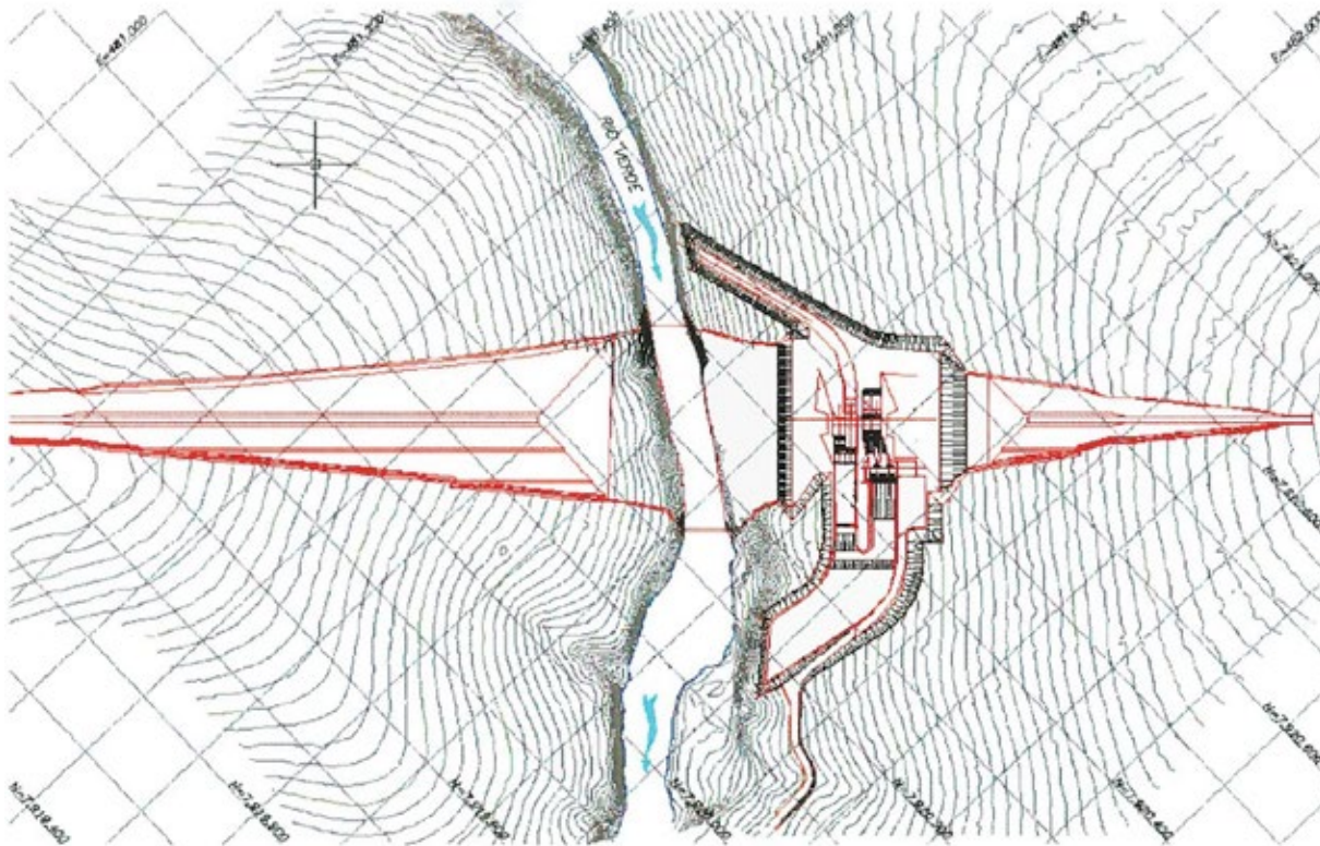
Figura 5. Desvio do rio feito em uma única fase. Construção das estruturas definitivas e galerias de desvio, a seco. UHE Salto, GO. Fonte: ROCHA, 2006
