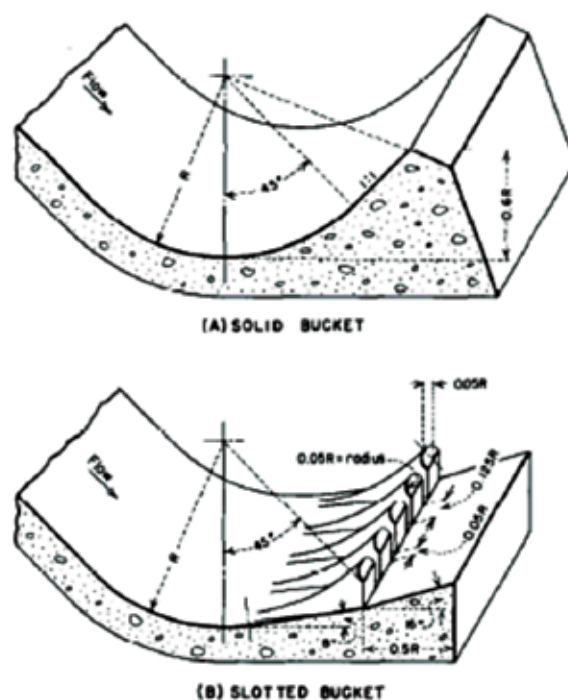
Figura 33. Bacia de dissipação do tipo roller bucket . Fonte: USBR, 1973
