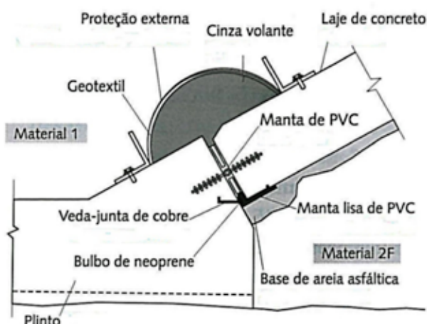
Figura 21. Junta perimetral. Utilização de cinza volante em alternativa ao mastique. Barragem de Aguamilpa, México.
