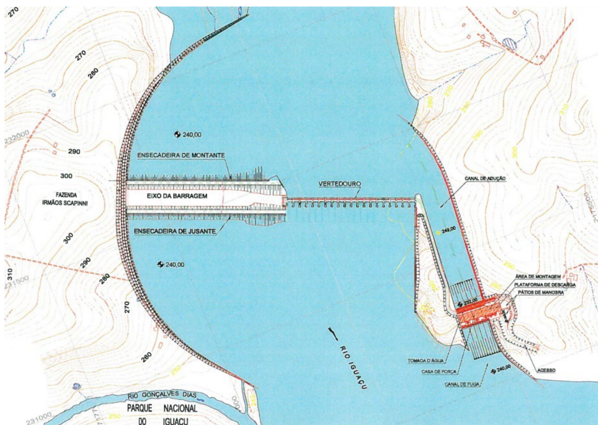
Figura 9. Desvio do rio em diversas fases. 2ª Fase. Desvio pelo vertedor, com uso de ensecadeira incorporada de montante e de jusante. UHE Baixo Iguaçu, PR.
