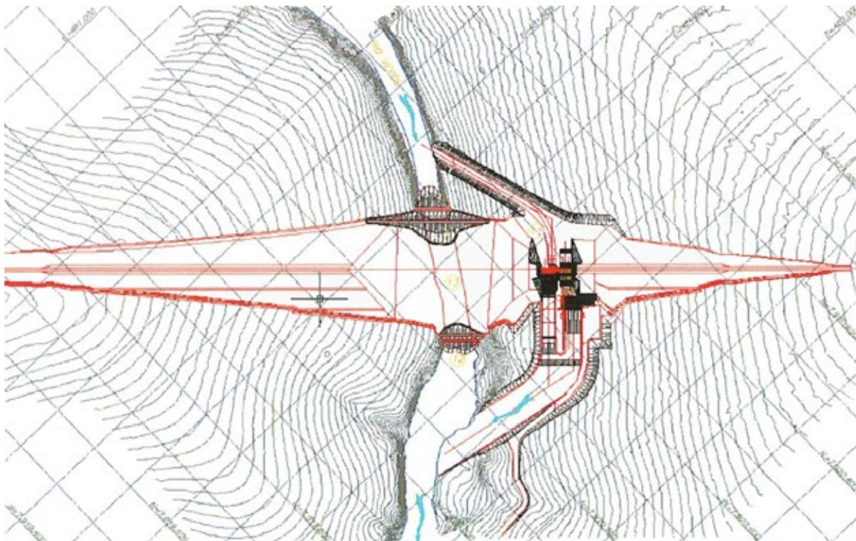
Figura 6. Desvio do rio feito em uma única fase. Desvio do rio feito pelas galerias de desvio. Leito ensecado com as ensecadeiras de montante e de jusante UHE Salto, GO. Fonte: ROCHA, 2006
