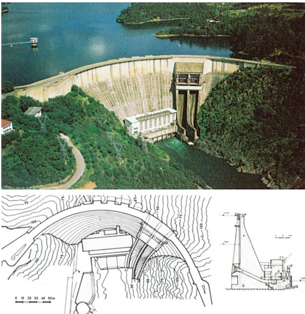
Figura 24. Barragem do Castelo do Bode, Portugal (arco-gravidade com 115 m de altura máxima, concluída em 1951).
