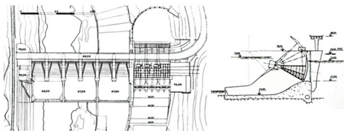
Figura 26. Barragem de Fratel, Portugal (barragem de soleira vertente, com 43 m de altura máxima, concluída em 1973).
