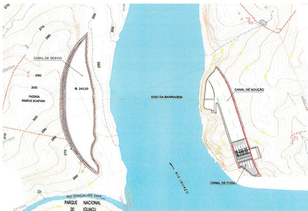
Figura 7. Desvio do rio em diversas fases. Escavação do canal de desvio na ombreira direita. UHE Baixo Iguaçu, PR. Fonte: ROCHA, 2006
