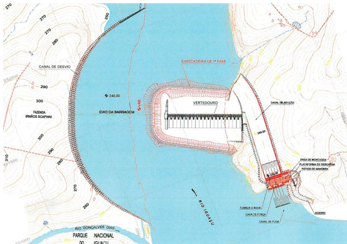
Figura 8. Desvio do rio em diversas fases. 1ª Fase. Desvio pelo leito estrangulado e canal lateral. UHE Baixo Iguaçu, PR. Fonte: ROCHA, 2006
