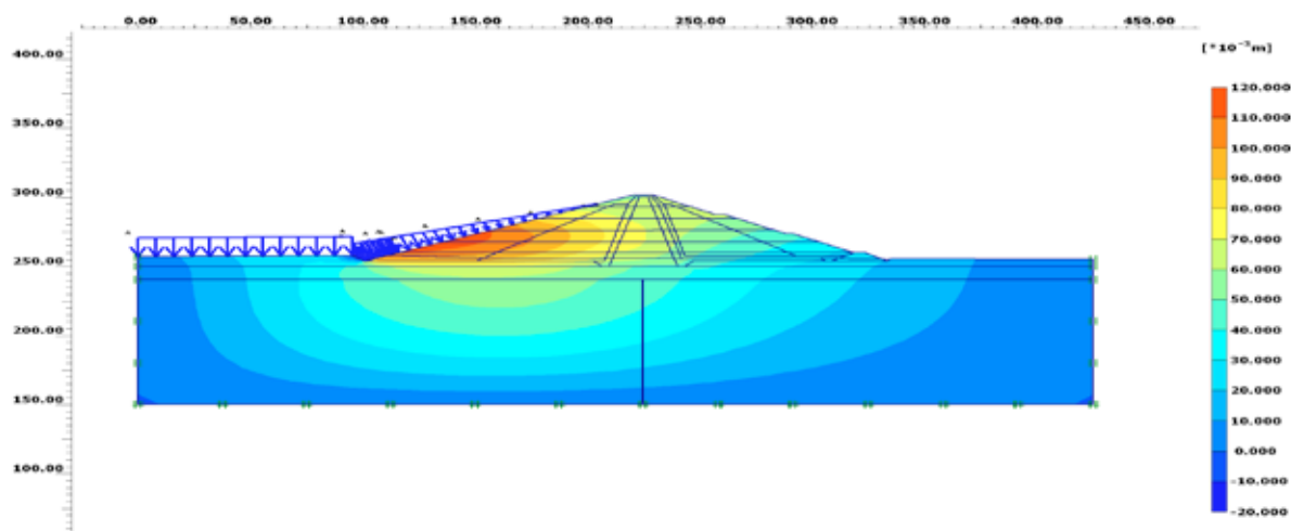
Figura 16. Análise de tensões deformações. Modelação do primeiro enchimento do reservatório. Deslocamentos horizontais.
