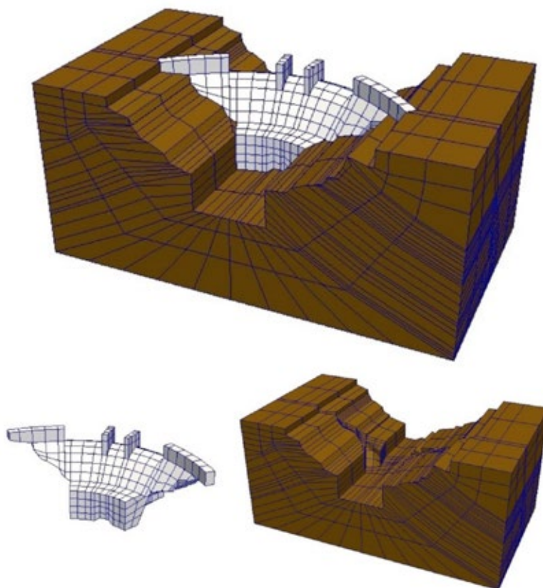
Figura 29. Modelo de elementos finitos de uma barragem de soleira vertente. Fonte: LNEC
