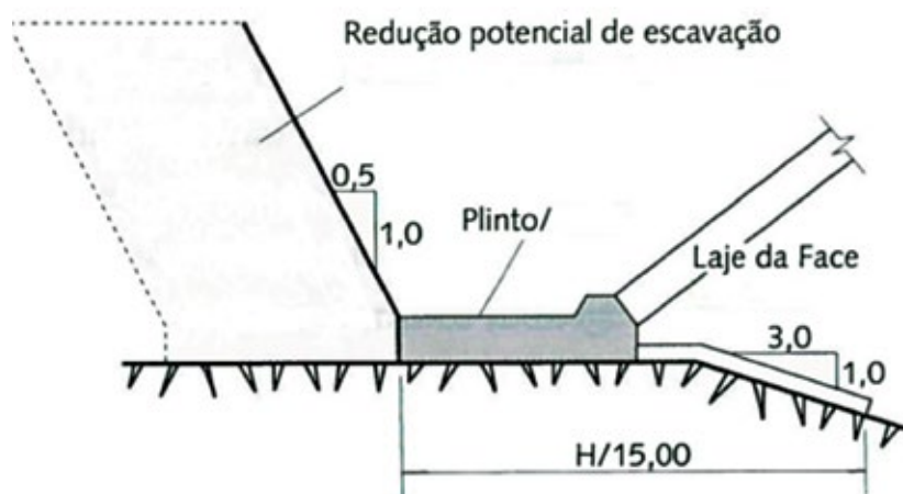
Figura 19. Seção da laje do plinto de montante e jusante (interno). Fonte: CRUZ; MATERÓN; FREITAS, 2009
