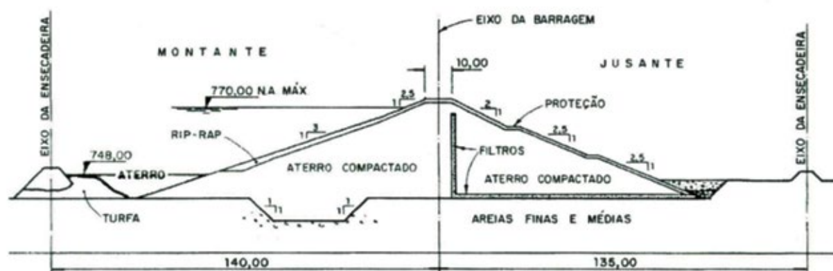
Figura 10. Seção típica de uma barragem de terra homogênea. Barragem de Ponte Nova, SP. Fonte: Cruz, 2004
