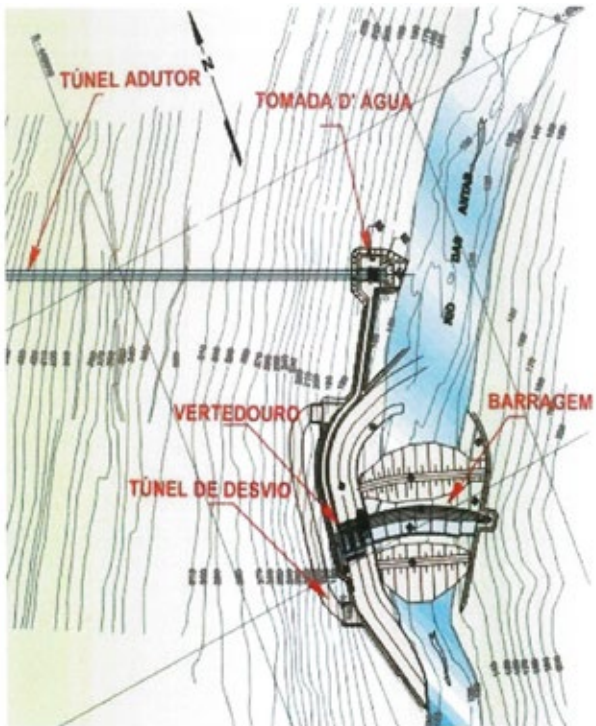
Figura 4. Desvio do rio por canal lateral na região do vertedor, associado a túnel de desvio. UHE Monte Claro, RS. Fonte: ROCHA, 2006
