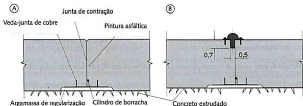
Figura 22. Juntas verticais: A) Campos Novos, área central (zona de compressão); B) Barra Grande, RS/SC, ombreiras (zona de tensão). Fonte: Cruz; Materón; Freitas, 2009
