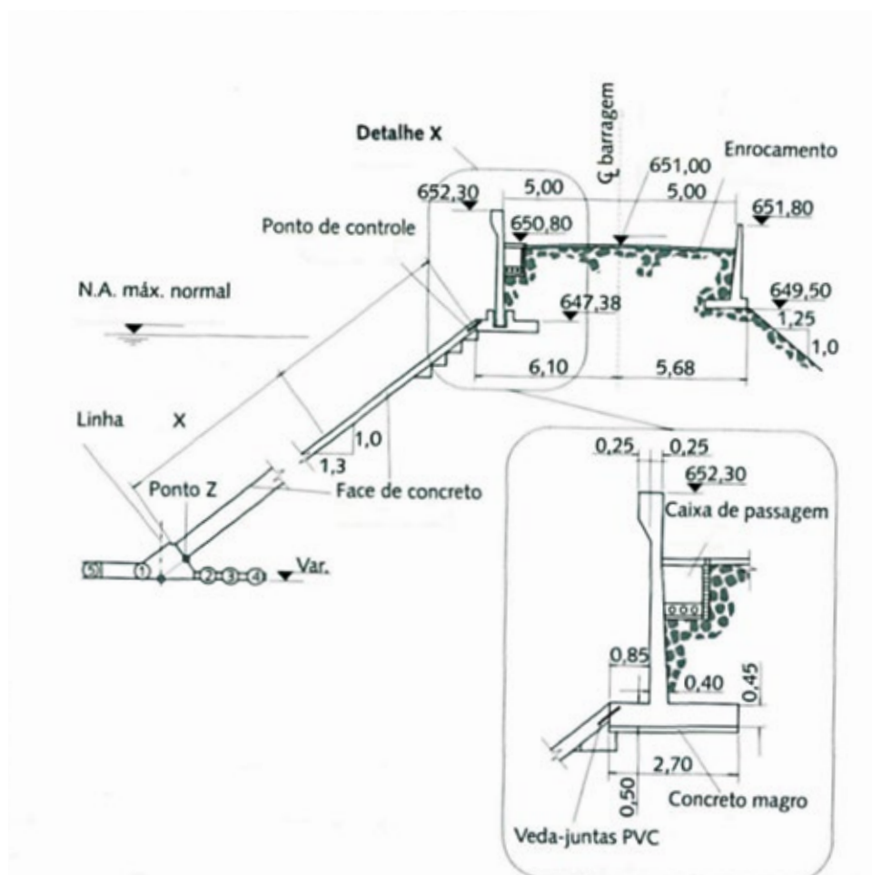
Figura 23. Detalhe do muro da crista e da junta de expansão no contato laje-fundação do muro da barragem de Barra Grande, RS/SC. Fonte: Cruz; Materón; Freitas, 2009
