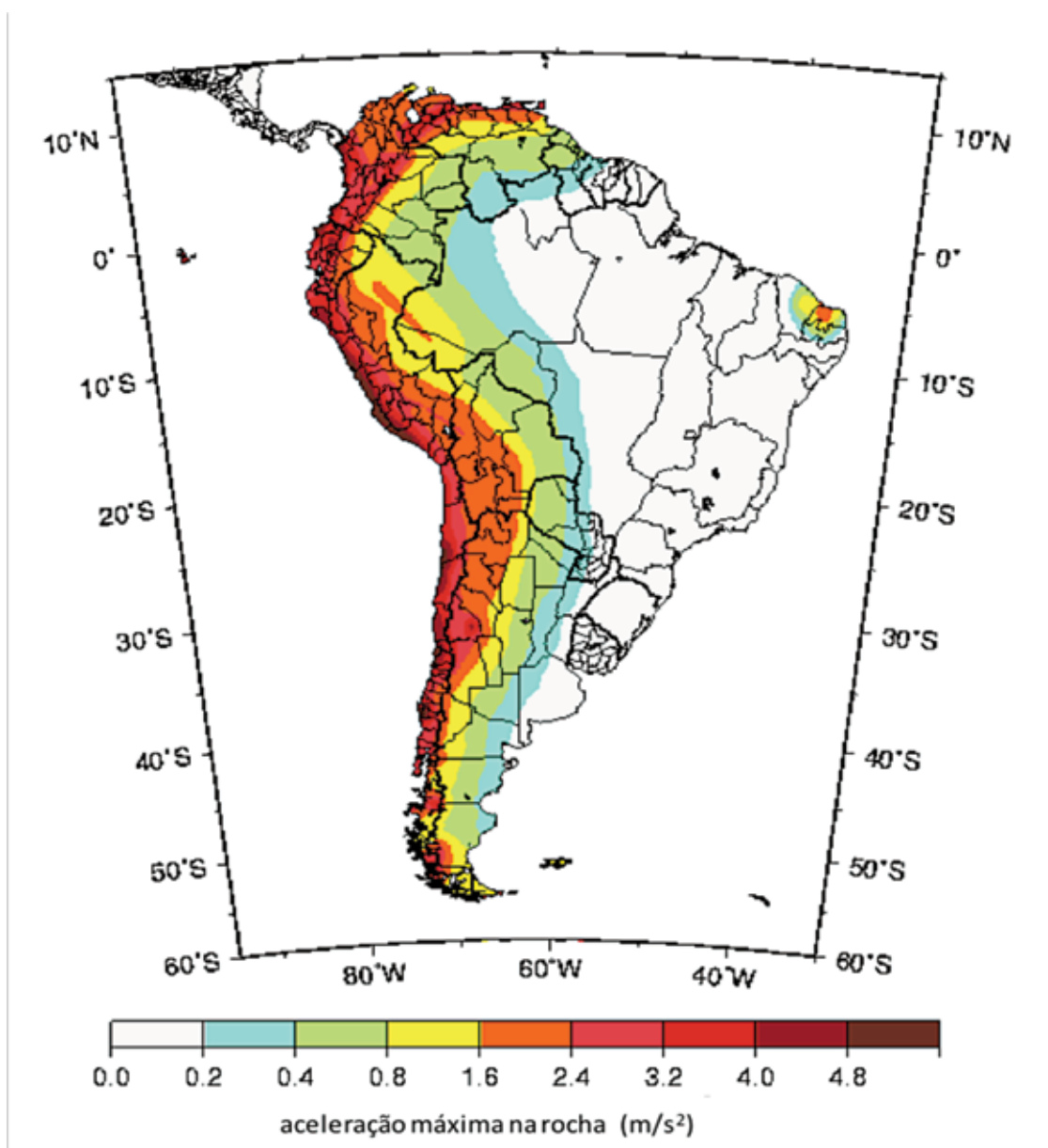
Figura 2. Mapa de risco sísmico na América do Sul. Aceleração máxima na rocha com a probabilidade de 90% de não ser excedida, para um período de 50 anos. Fonte: GSHAP
