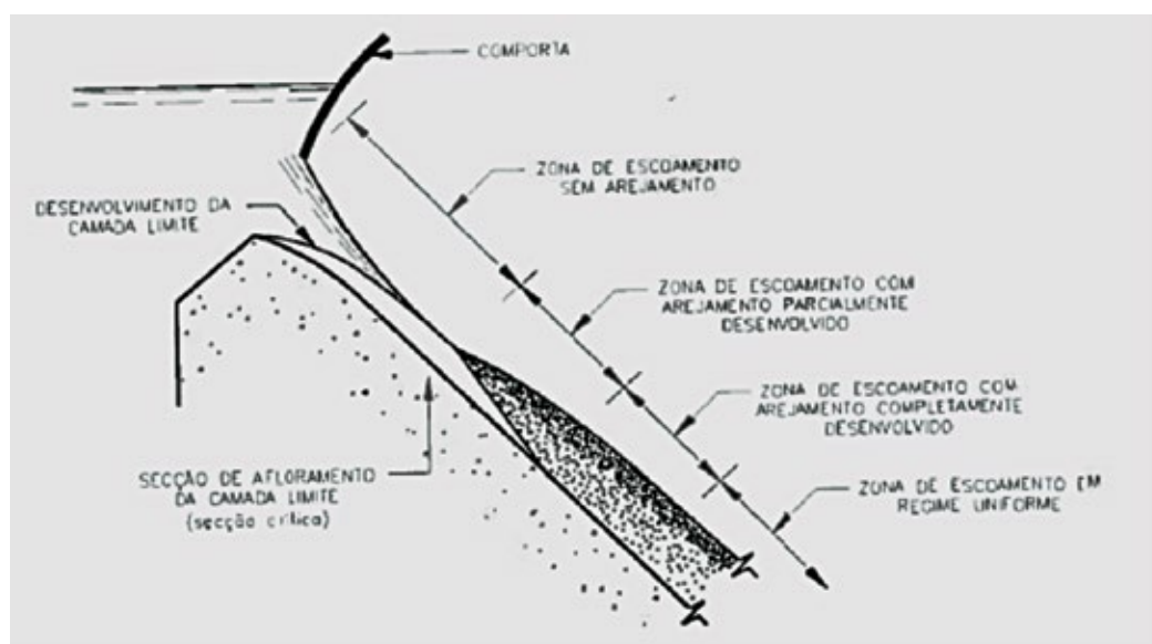
Figura 38. Regimes de escoamento a jusante de uma comporta. Fonte: INAG, 2001
