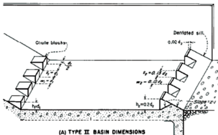
Figura 32. Bacia de dissipação do Tipo II. Fonte: USBR, 1973
