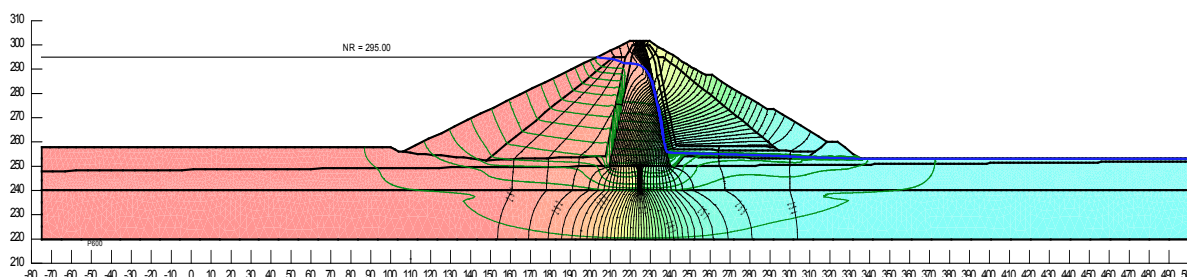
Figura 14. Análise de percolação em regime permanente pelo método dos elementos finitos (linhas equipotenciais).
