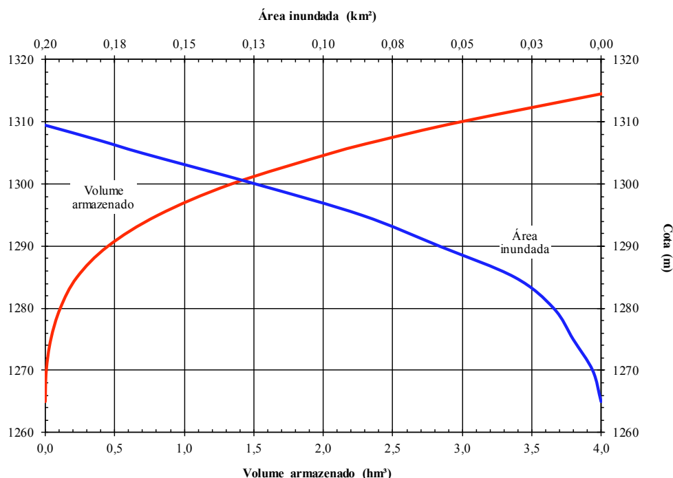
Figura 41. Exemplo de curvas de áreas inundadas e volumes armazenados de um reservatório. Fonte: COBA, S.A.
