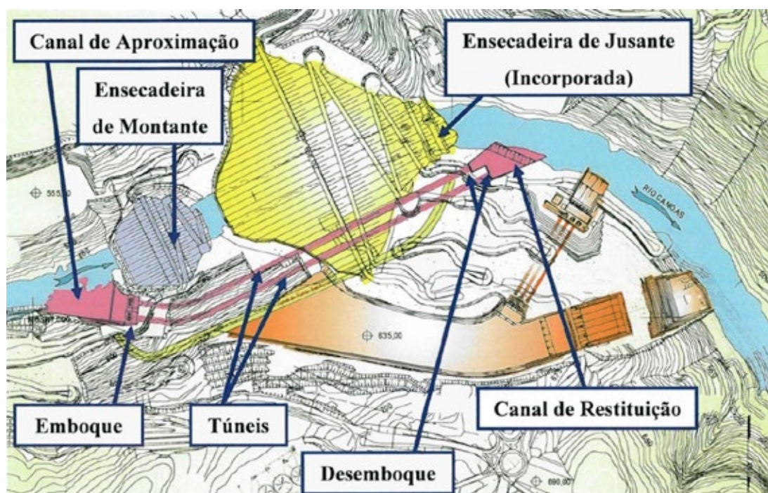
Figura 3. Estruturas do sistema de desvio de rio por túnel. UHE Campos Novos, SC. Fonte: ROCHA, 2006
