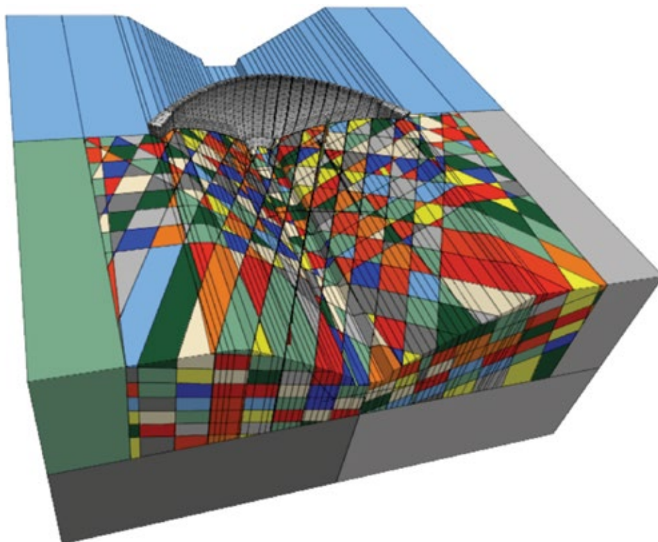
Figura 28. Modelo de elementos finitos (barragem) e de elementos discretos (maciço rochoso de fundação) utilizado no estudo de uma barragem em arco. Fonte: LNEC
