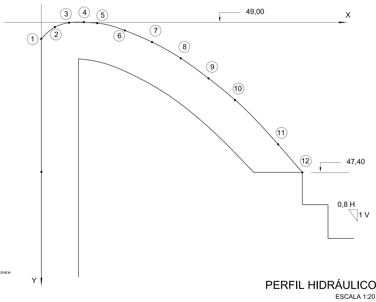
COORDENADAS DO PERFIL HIDRÁULICO
