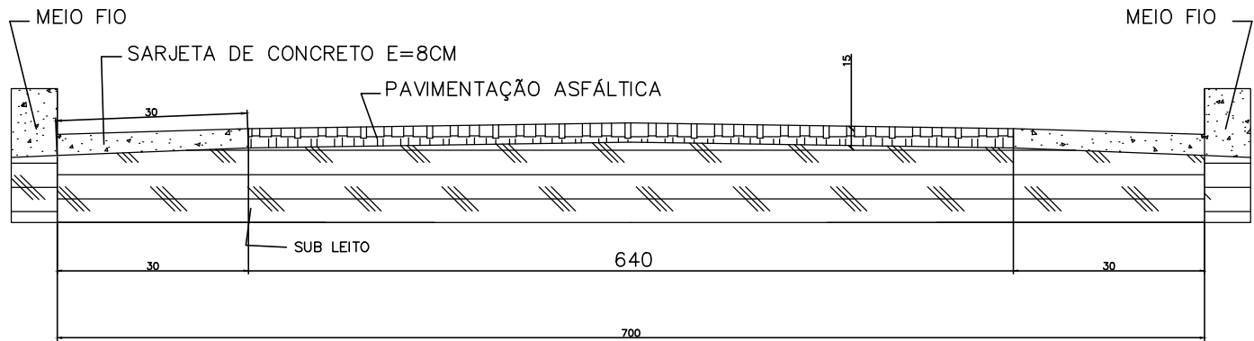
SEÇÃO TRANSVERSAL DA VIA SEM ESCALA
