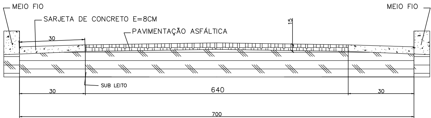
SEÇÃO TRANSVERSAL DA VIA SEM ESCALA
