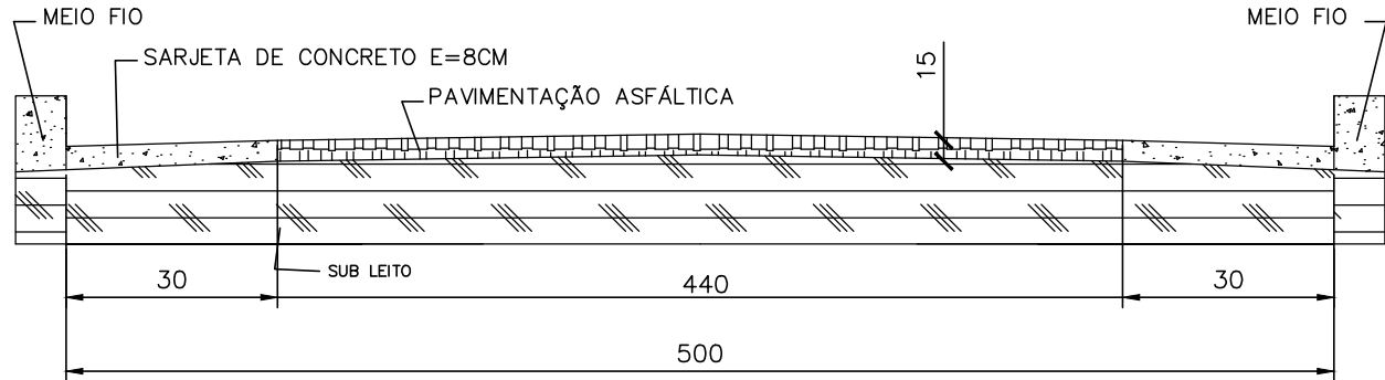
SEÇÃO TRANSVERSAL DA VIA SEM ESCALA
